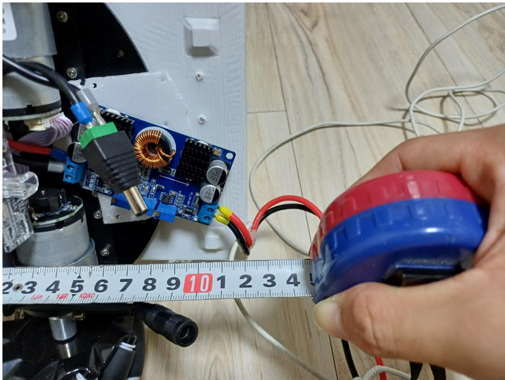
보드에서 TopRight 외곽까지의 길이. 121mm이다.
