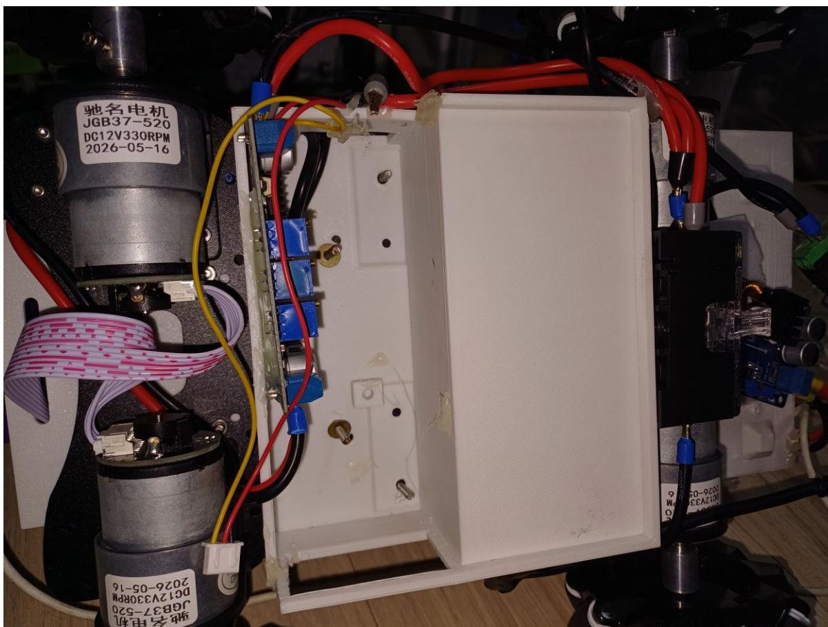
나사 제거한 모습. 나사가 체결된 4개의 위치.
