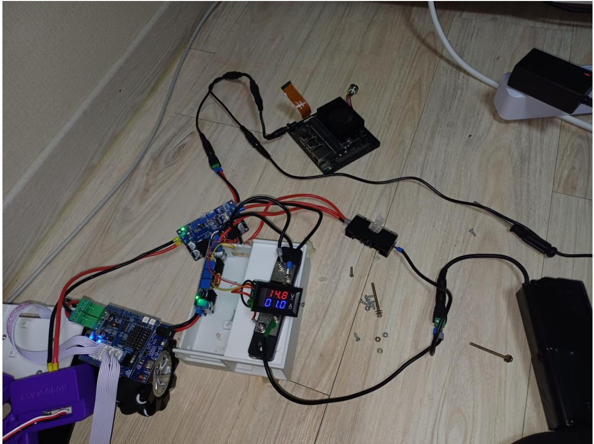
전원 계통
