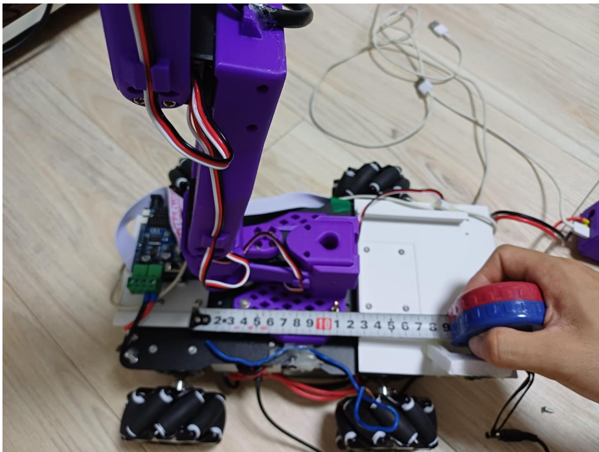
두 보드간 나사 실측 장면
